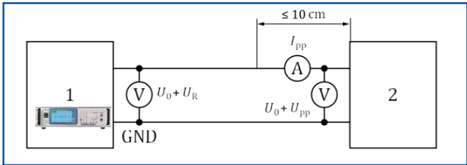
图5- 交流电压的测试设置 1: HY-BP系列汽车电子测试高速电源 2: 被件件 U R : 电源处的交流纹波电压 U pp : 交流峰值电压 U 0 : 施加的试验电压的直流电平, 单位为伏特 I pp : 交流峰值电流 电压表和电流表与被件件的距离在10cm以内。
